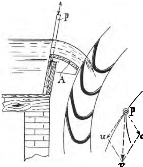
Fig. 17. Überfallwehrrad bei einem rückschlächtigen Wasserrad.
